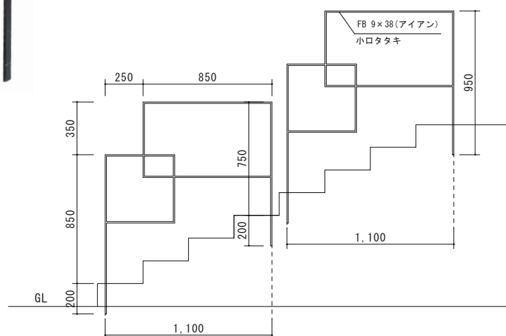
階段手摺
