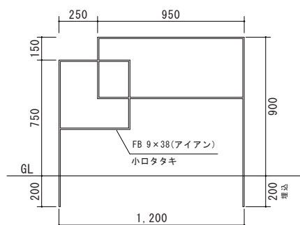
水平手摺
